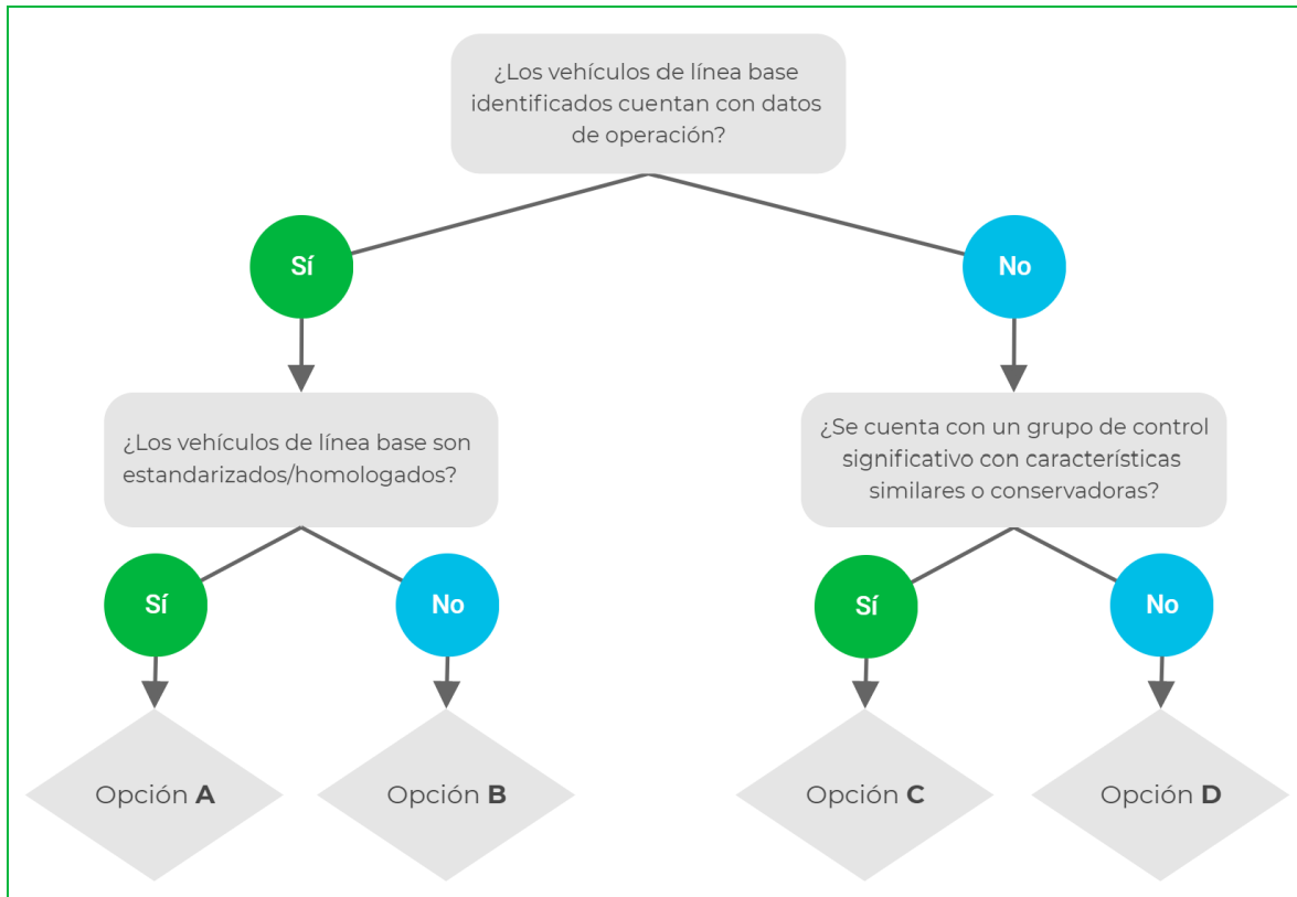
Gráfico 4. Árbol de decisión para determinar la eficiencia de un combustible en un vehículo de línea base.
